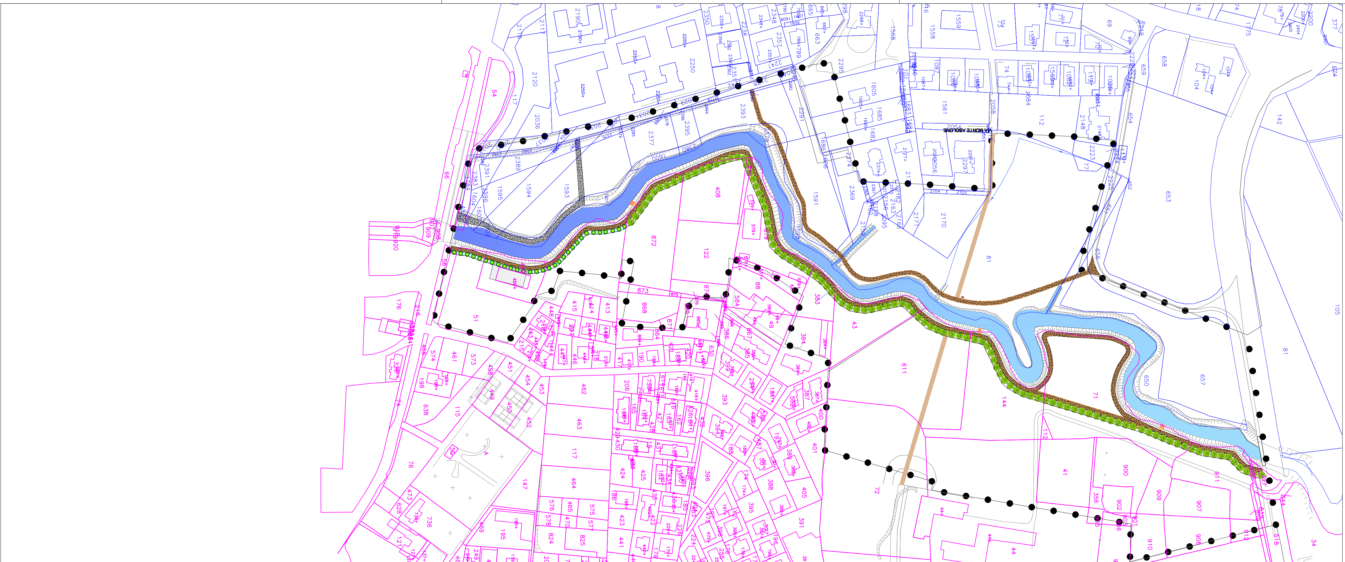
SOVRAPPOSIZIONE CATASTALE-PROGETTO
